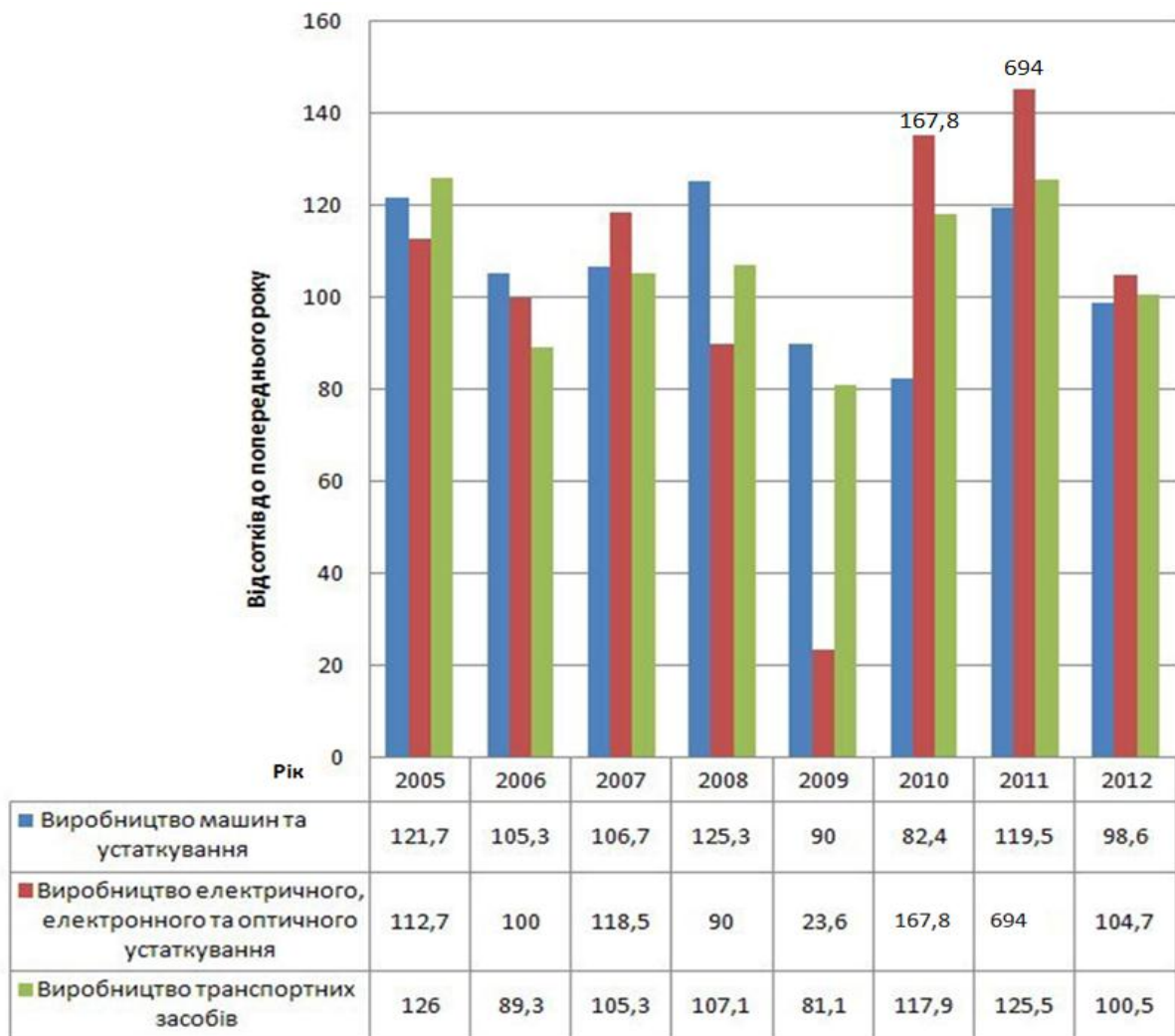
Рис. 3. Динаміка випуску продукції машинобудування за видами діяльності (побудовано за даними [4])
