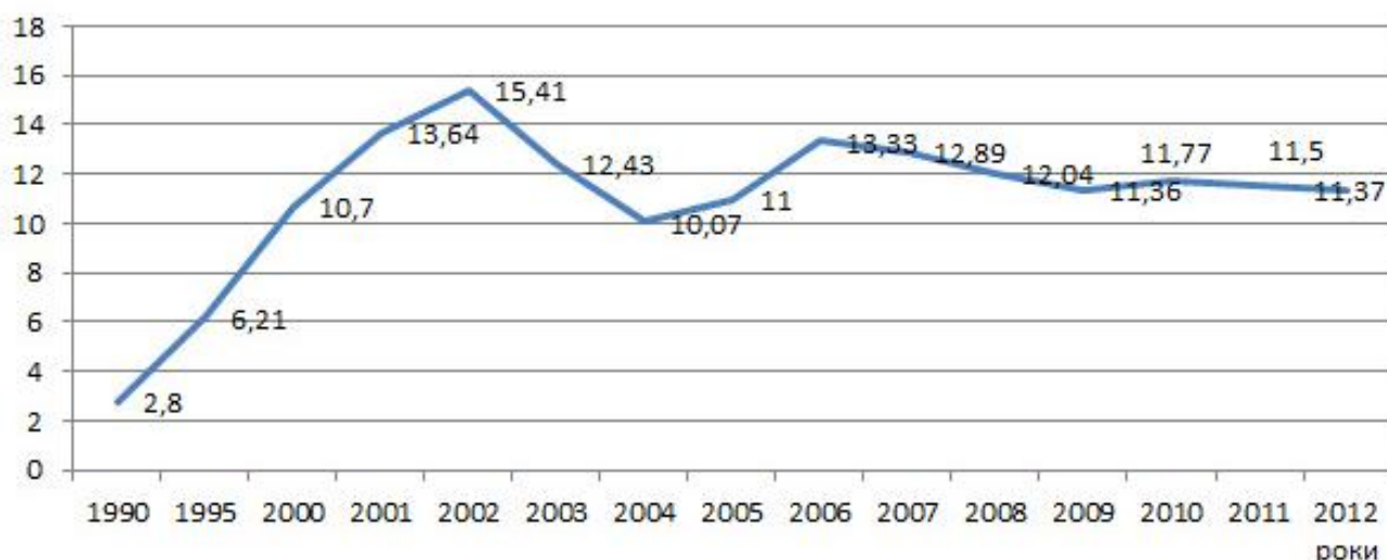
Рис. 3. Втрати води при транспортуванні, млн. м³
