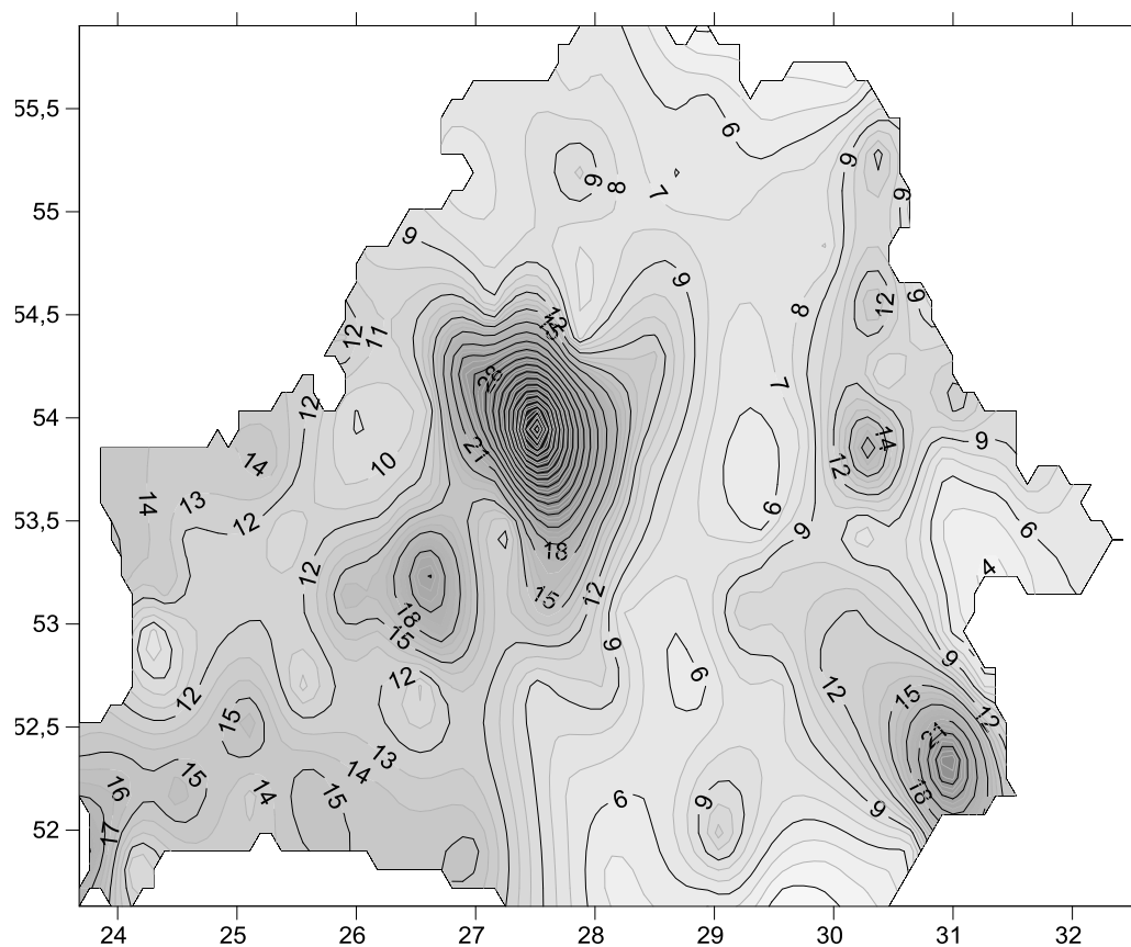
Рис. 4. Карта изолиний плотности сельского населения, составленная по значениям плотности в центральной точке административных районов
